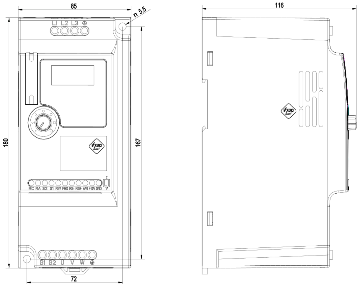
Rozmerový výkres A550 PLUS - 4kW 4T0040
